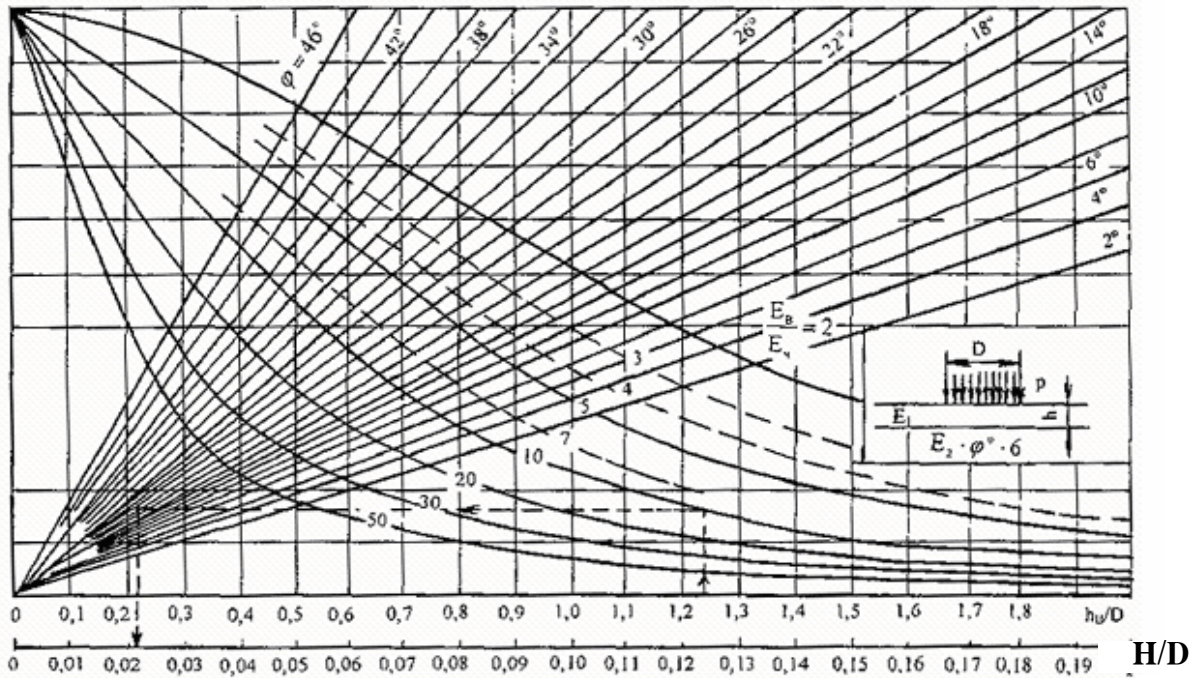
Hình 3-2: Toán đồ xác định ứng suất trượt từ tải trọng bánh xe ở lớp dưới của hai lớp ( H/D = 0 \div 2,0 )
