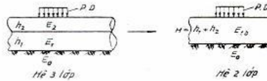
Hình 3-2: Sơ đồ đổi hệ 3 lớp về hệ 2 lớp (Các lớp ký hiệu số thứ tự tăng dần từ dưới lên)
