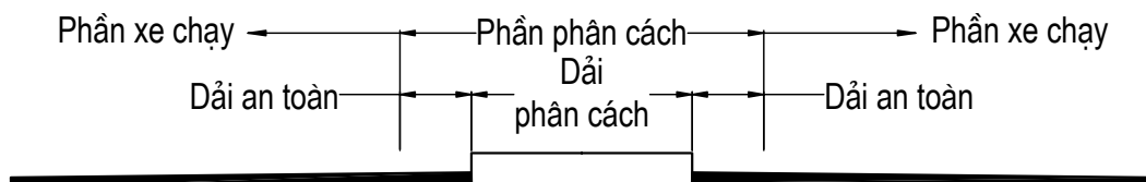
Hình 4. Cấu tạo điển hình phân phân cách
