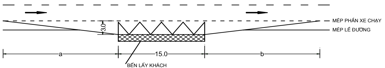
Hình 13 . Cấu tạo chỗ dừng xe có làn phụ, dạng dừng tránh.
